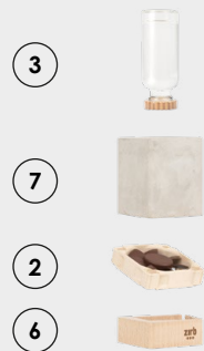
zirb.Minimal
